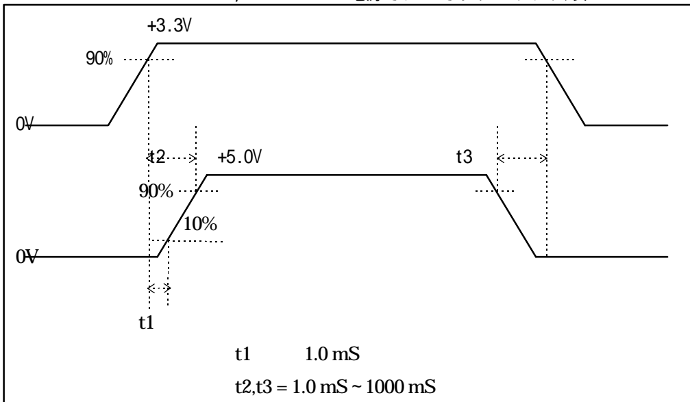
+5.0V、+3.3V 電源オン/オフシーケンス表
